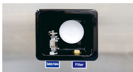
역류방지 공기순환필터
